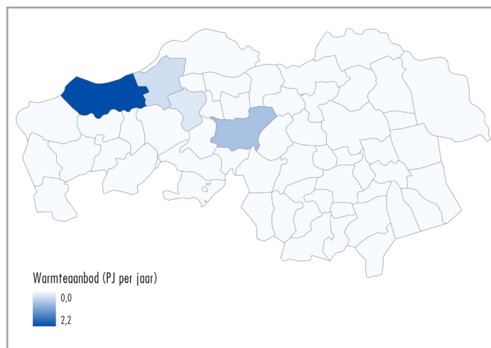
Kaart 42 – Verwacht aanbod geothermie 2050
