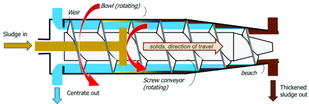
Figuur 16 Decatercentrifuge
