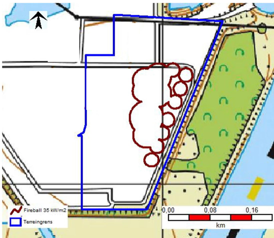
Figuur 29 Explosieaandachtsgebied
