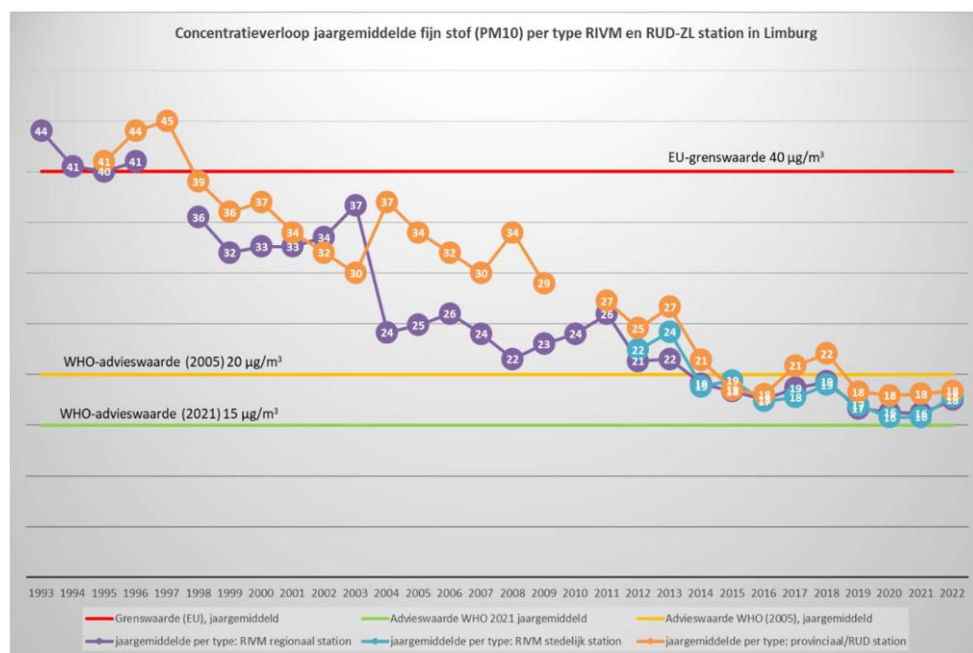
Figuur 27 Jaargemiddelden PM 10 , afname 1993-2022
