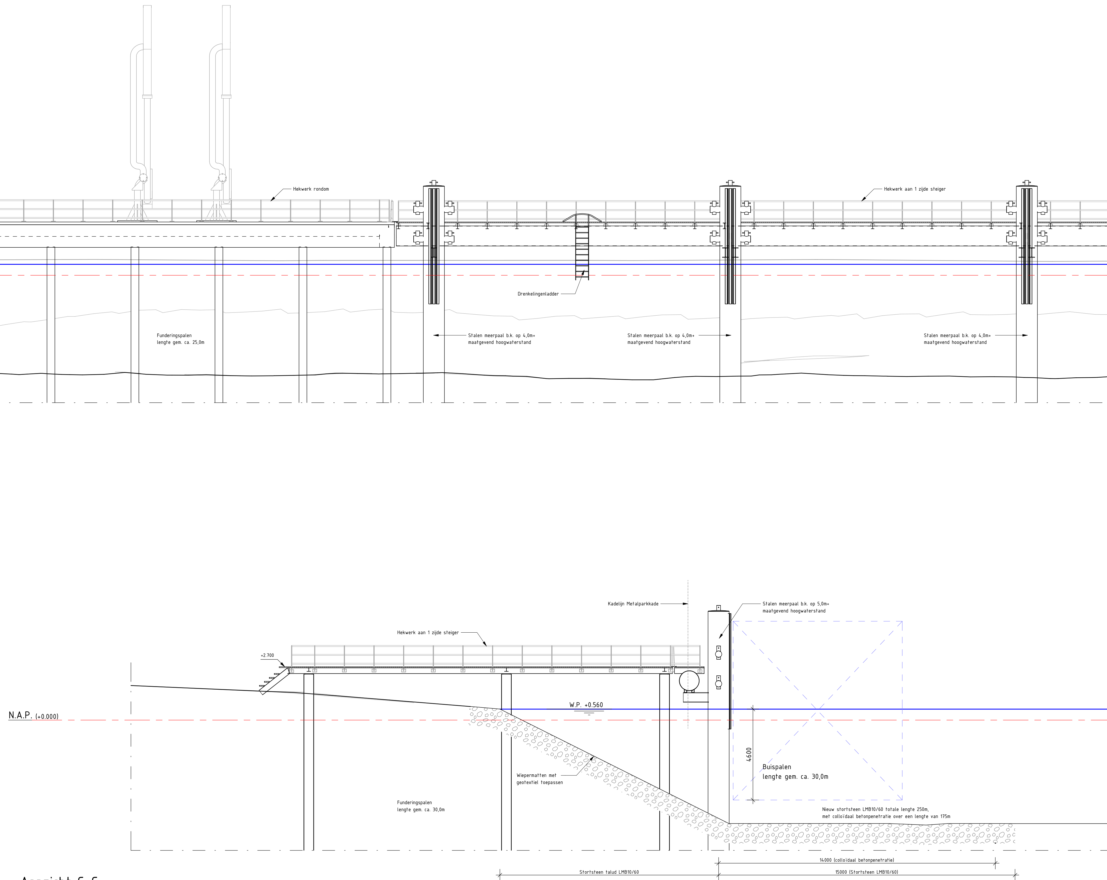
Aanzicht C-C Schaal: 1 : 100
