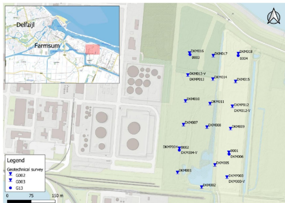
Figuur 3.1 Grondonderzoekspunten
